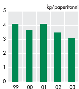
Paperitehtaiden jätevesien kemiallinen hapen kulutus (COD) 1)
