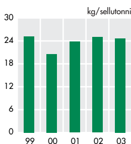
Sellutehtaiden jätevesien kemiallinen hapen kulutus (COD)
