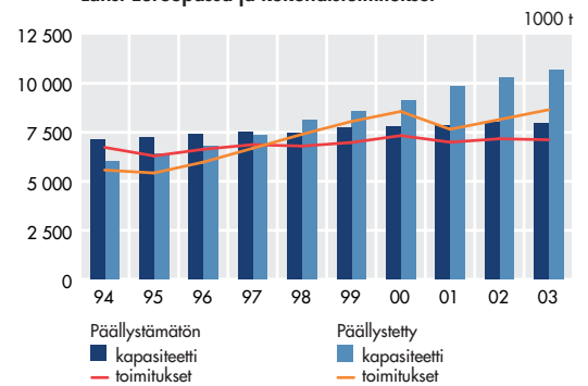
Hienopaperin tuotantokapasiteetit Länsi-Euroopassa ja kokonaistoimitukset
