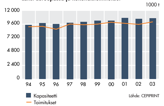
Sanomalehtipaperin tuotantokapasiteetit Länsi-Euroopassa ja kokonaistoimitukset
