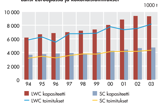
Aikakauslehtipaperin tuotantokapasiteetit Länsi-Euroopassa ja kokonaistoimitukset
