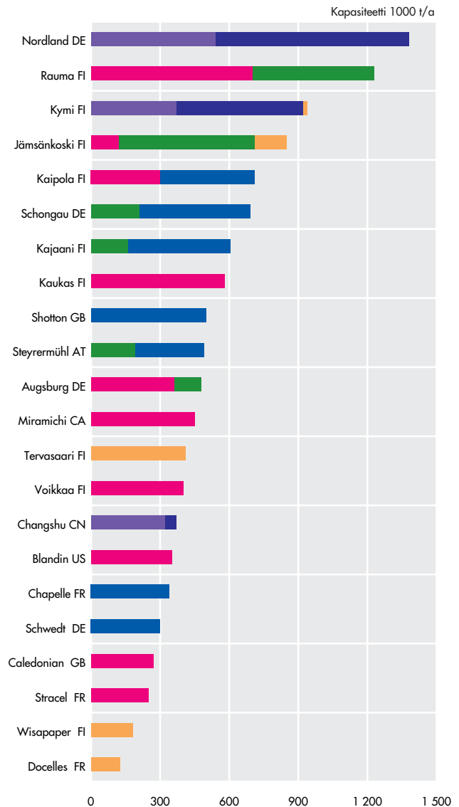
Tuotantokapasiteetit tehtaittain tammikuussa 2004
