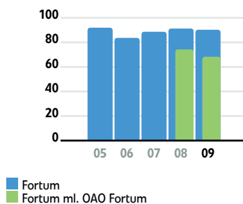
CO 2 -päästöttömien energianlähteiden osuus sähkön tuotannossa, %
