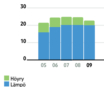
Divisioonan kaukolämmön ja höyryn myynti, TWh
